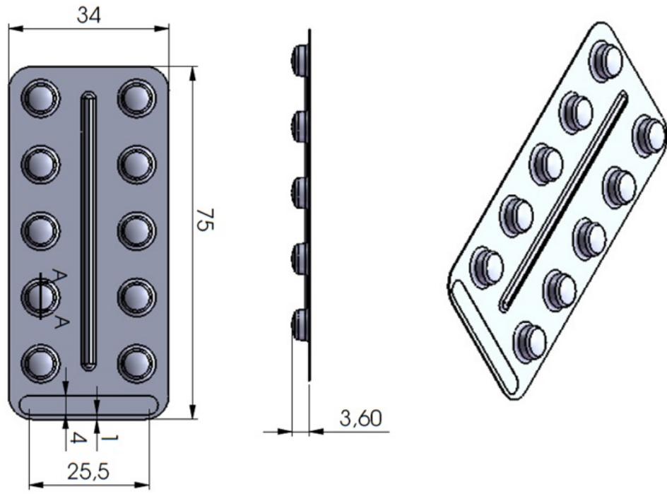
Desenho e dimensões do blister
